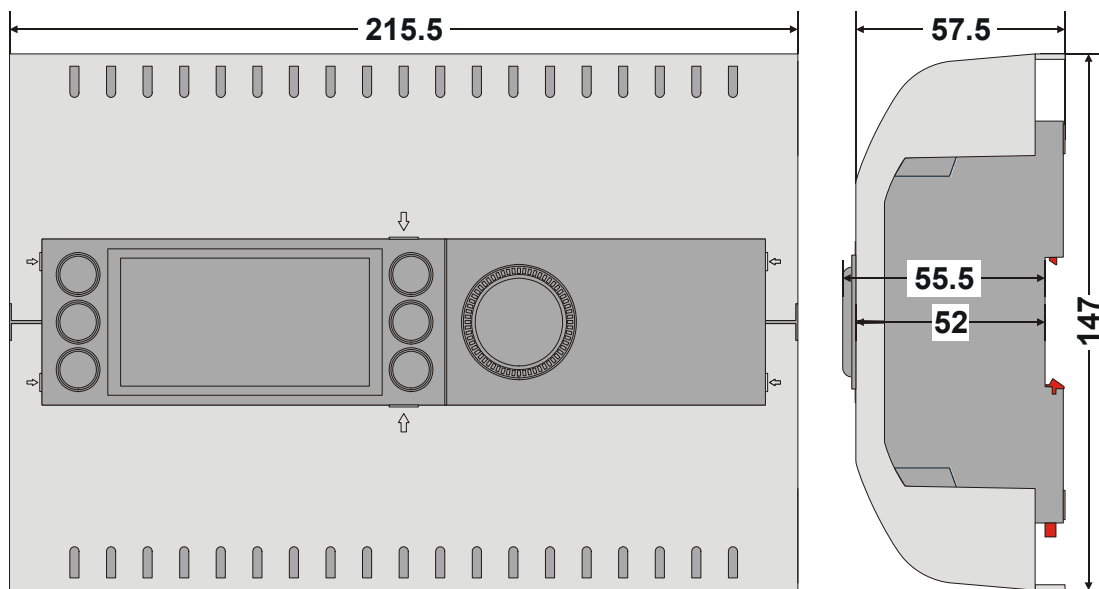
Размеры контроллера MVC с дополнительными крышками AC1 (в мм.)
